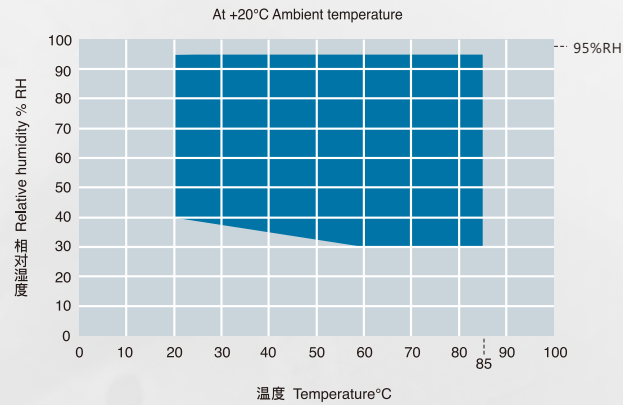
溫度控制範圍梯形圖
